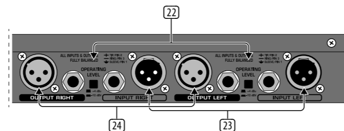
Fig. 3.6: Conexiones en la parte trasera del FBQ2496
