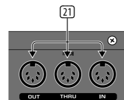
Fig. 3.5: Conexiones MIDI del FBQ2496
