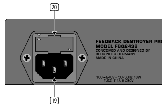
Fig. 3.4: Conexión a red eléctrica, fusible y número de serie
