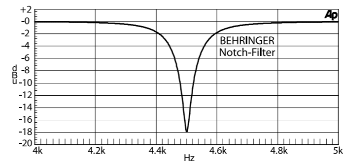
Fig. 4.1: Curva de un filtro muy estrecho
