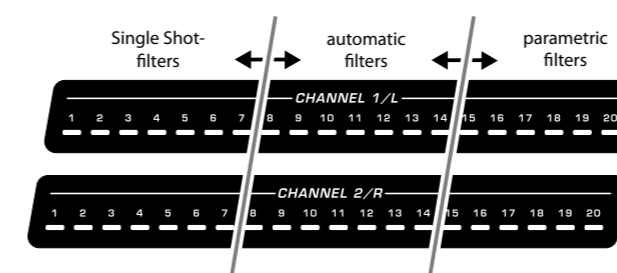
Fig. 4.2: Tipos de filtro del FBQ2496 (en estéreo, en este caso)
