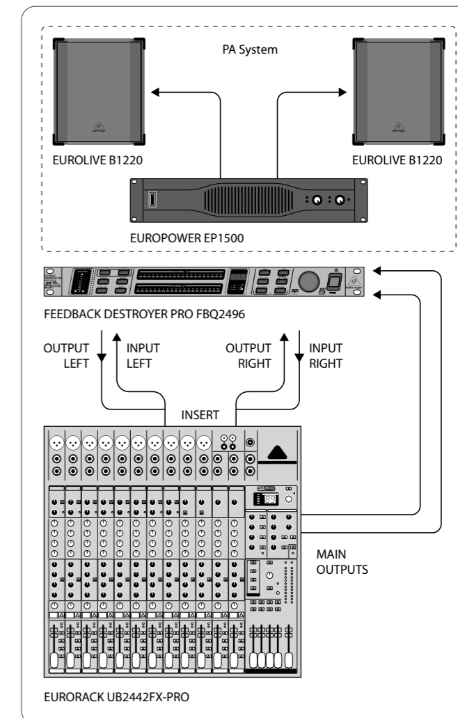
Fig. 5.2: El FEEDBACK DESTROYER PRO insertado en un canal y un subgrupo
