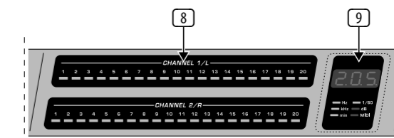
Fig. 3.2: Indicadores de estado y nivel del FBQ2496
