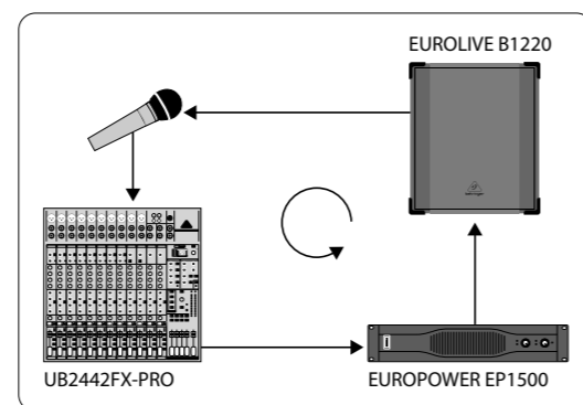
Fig. 2.1: Bucle de masa
