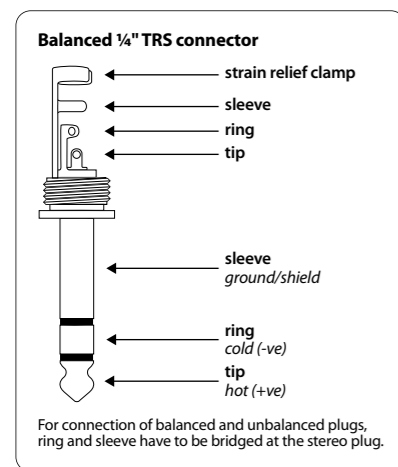
Fig. 8.1: Jack estéreo de 6,3 mm
