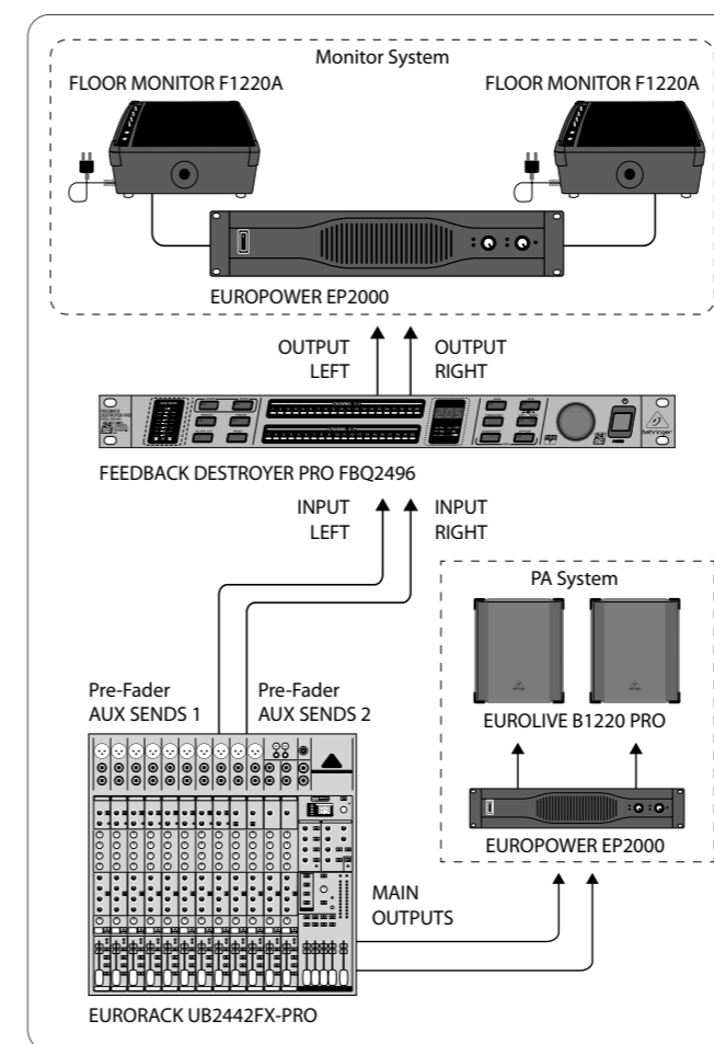
Fig. 5.1: Conexión del FBQ2496 para monitorización
